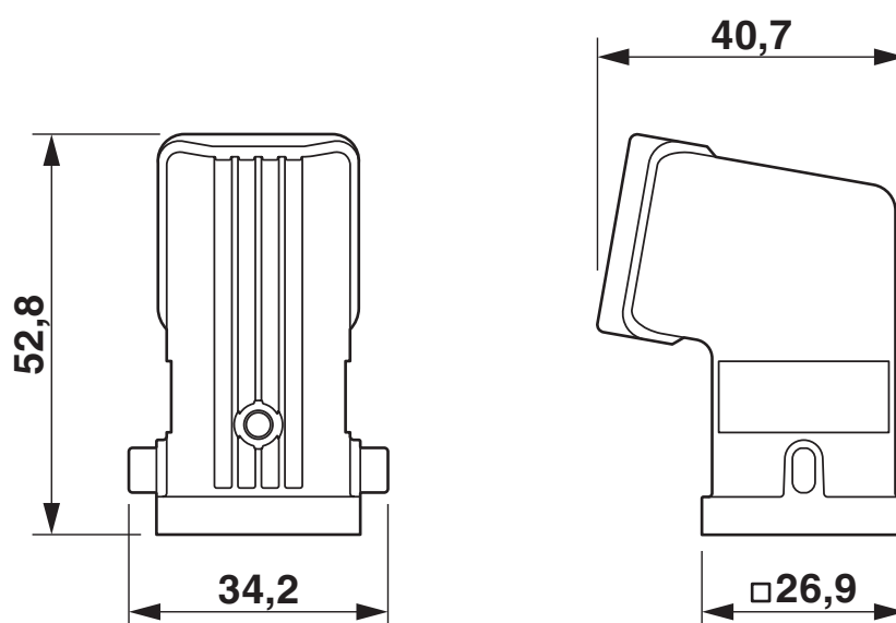
Rysunek wymiarowy
