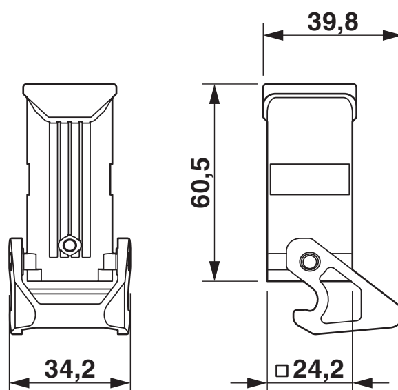
Rysunek wymiarowy
