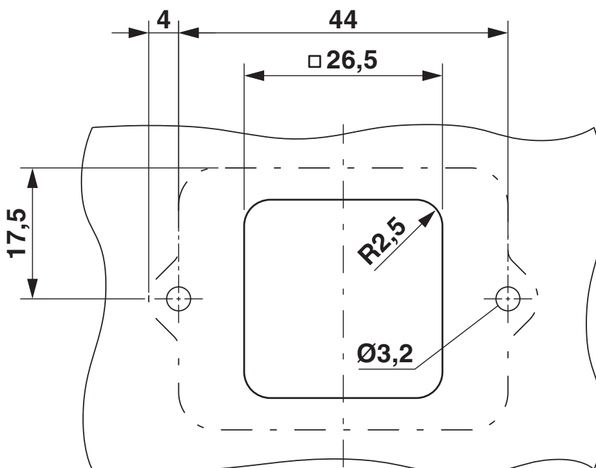
Rysunek wymiarowy
