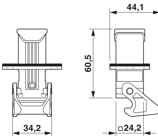
Rysunek wymiarowy
