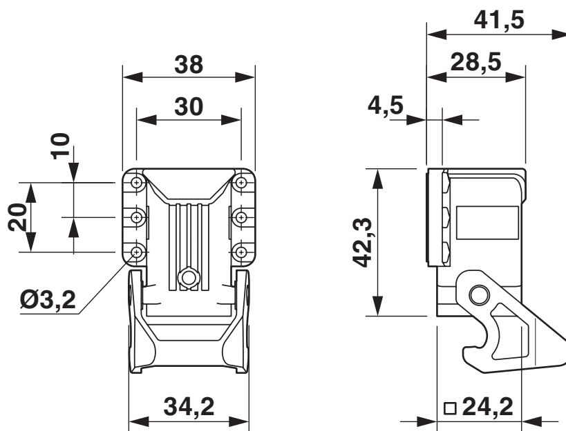
Rysunek wymiarowy
