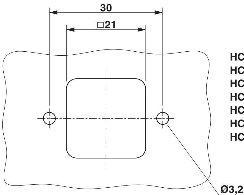
Rysunek wymiarowy
