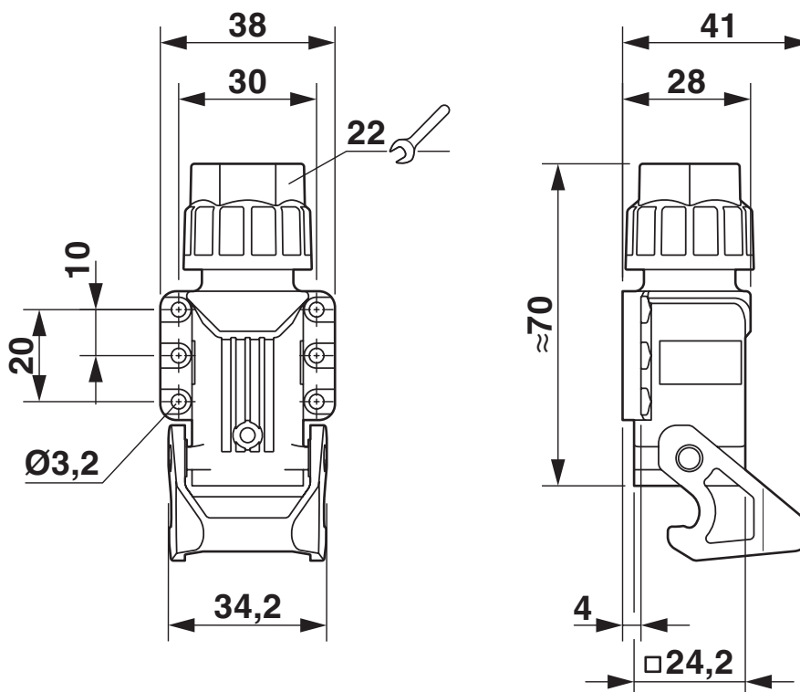
Rysunek wymiarowy
