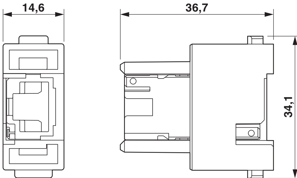
Rysunek wymiarowy
