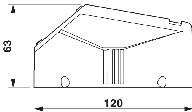
Rysunek wymiarowy
