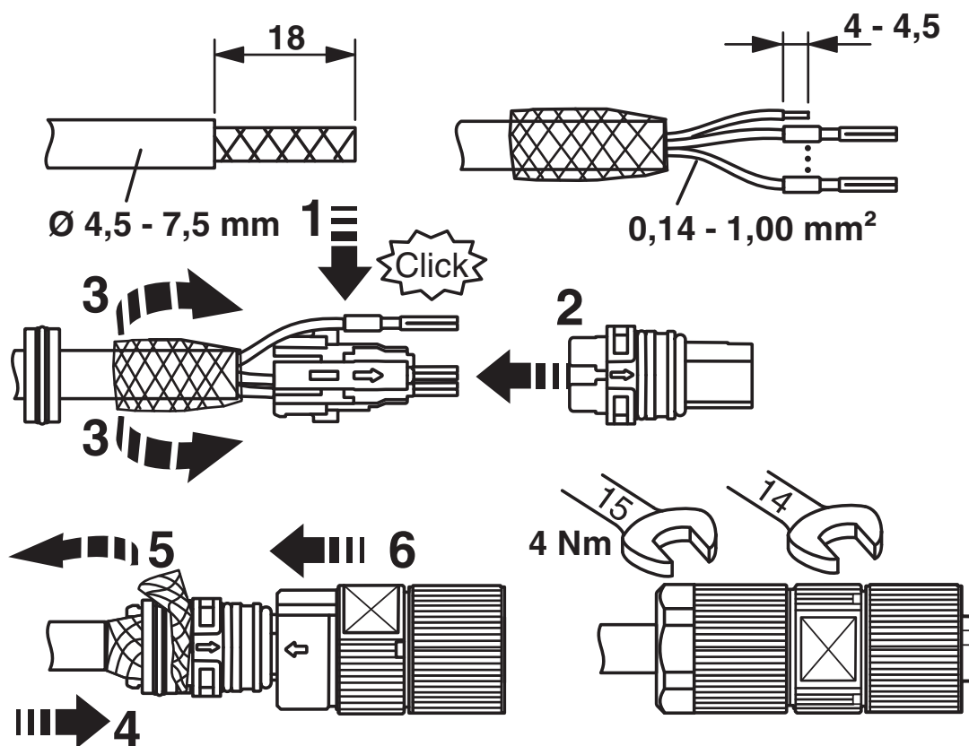
rysunek funkcyjny
