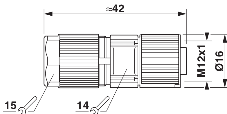
Rysunek wymiarowy
