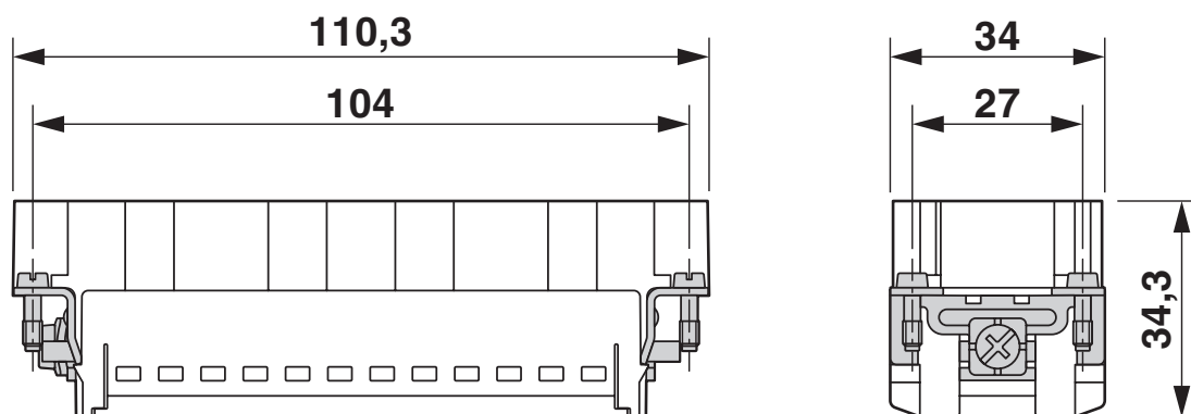
Rysunek wymiarowy
