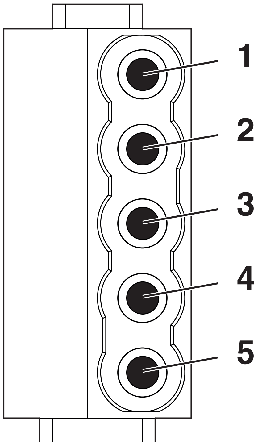
Rysunek schematyczny
