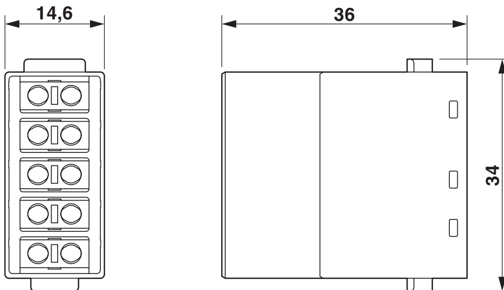
Rysunek wymiarowy
