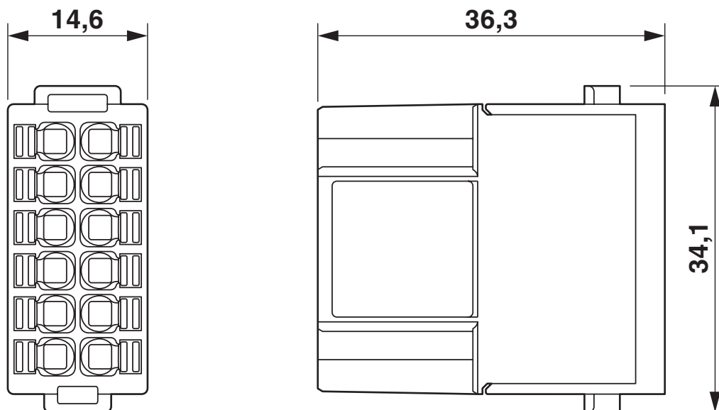
Rysunek wymiarowy
