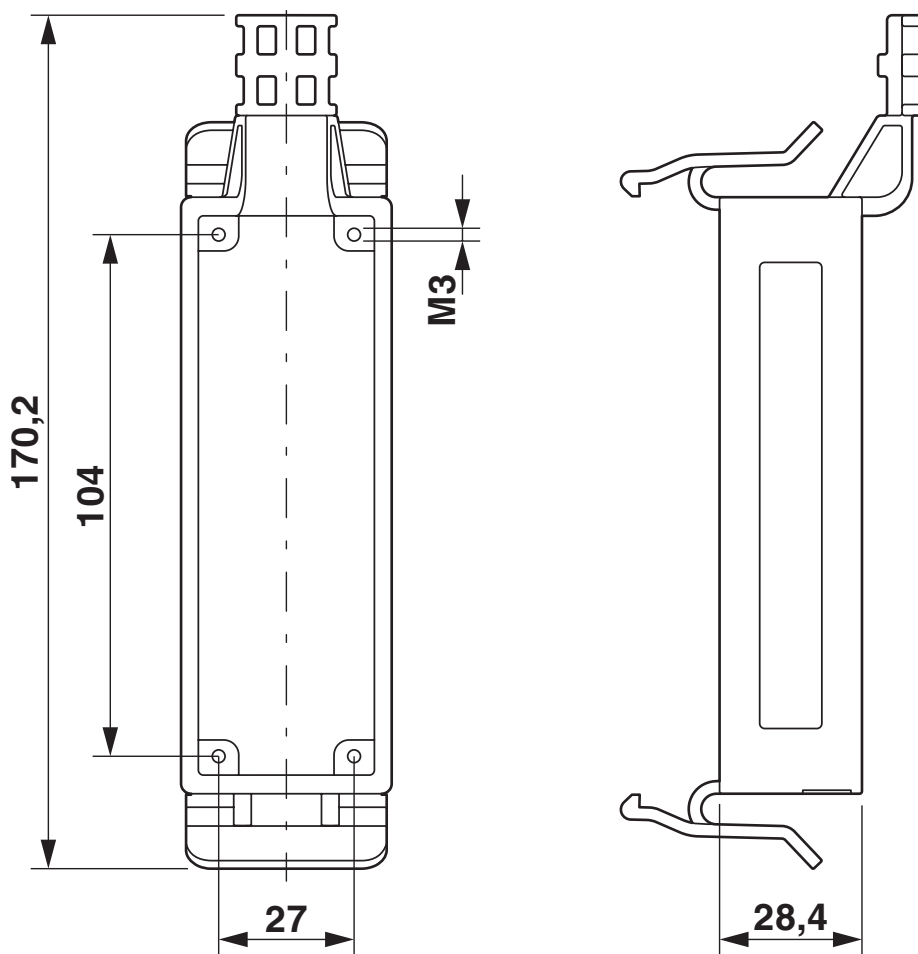
Rysunek wymiarowy
