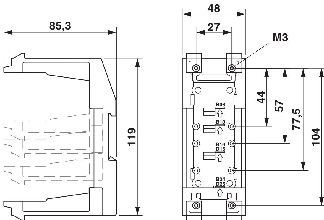
Rysunek wymiarowy
