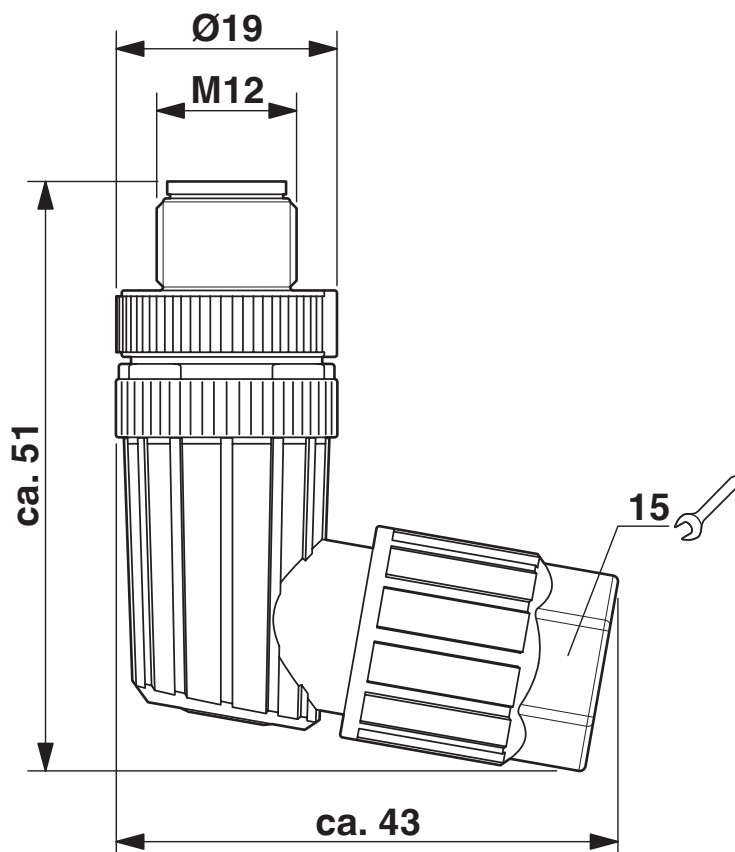
Rysunek wymiarowy
