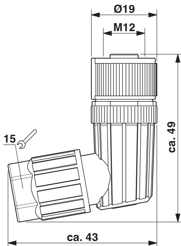
Rysunek wymiarowy
