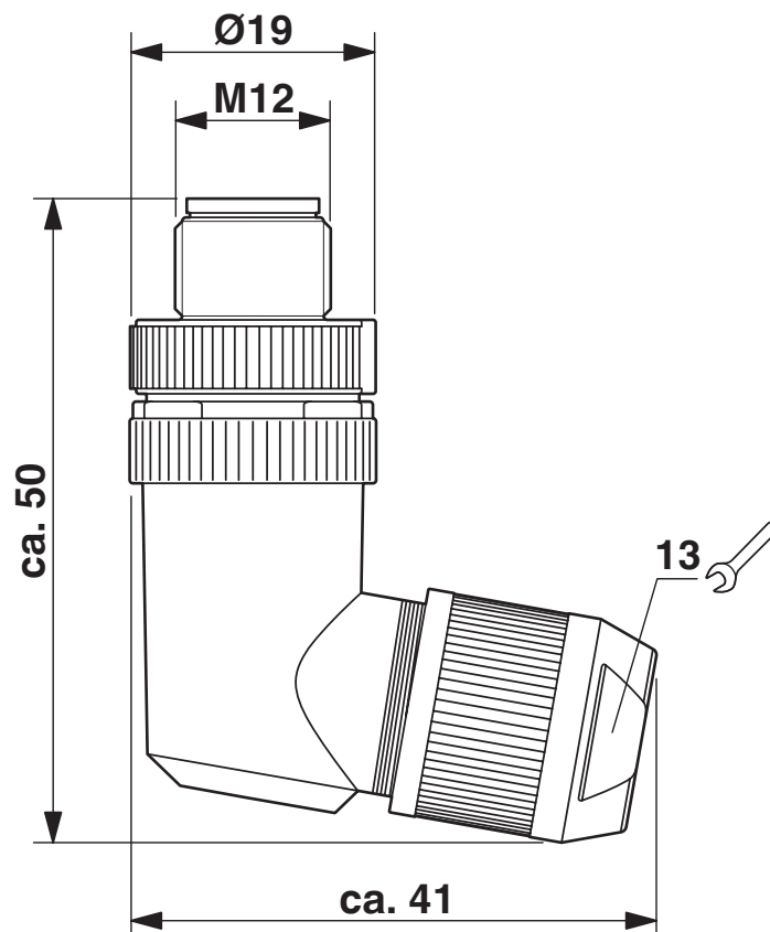
Rysunek wymiarowy
