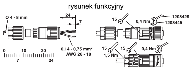
Rysunek schematyczny
