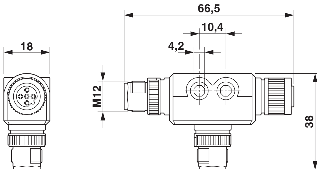
Rysunek wymiarowy
