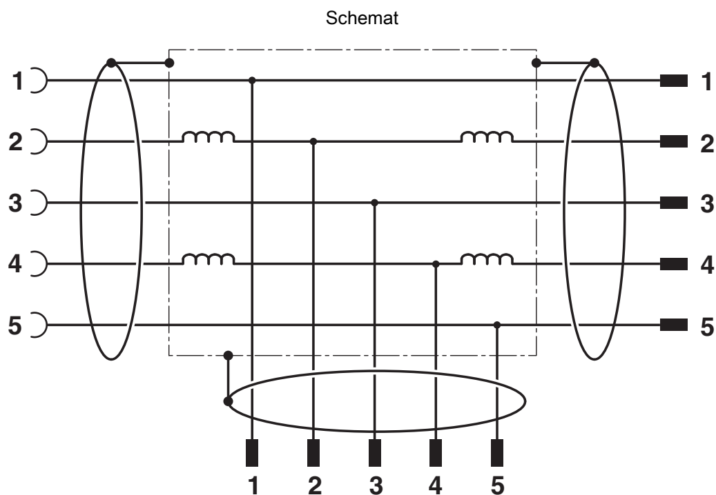
Rysunek schematyczny
