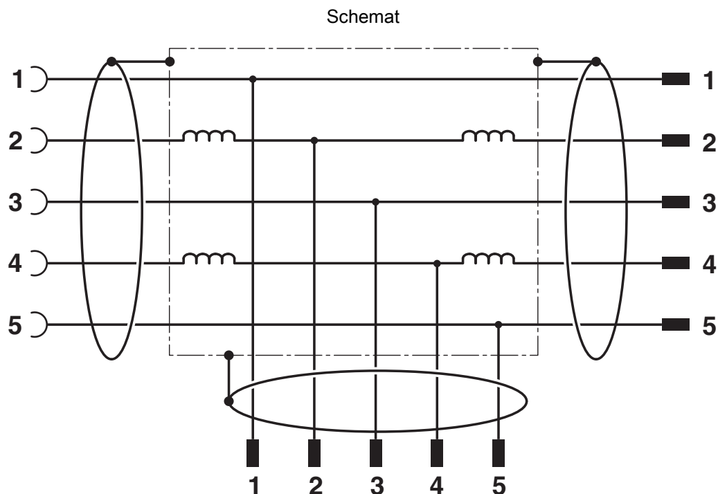
Rysunek schematyczny
