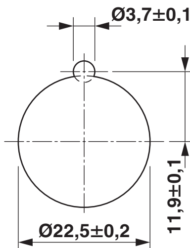
Rysunek wymiarowy
