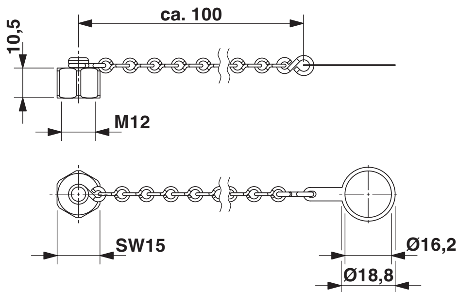
Rysunek wymiarowy
