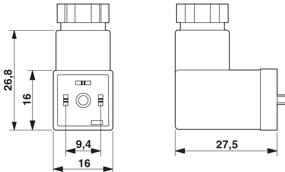
Rysunek wymiarowy
