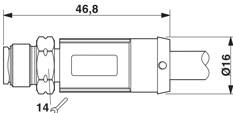
Rysunek wymiarowy
