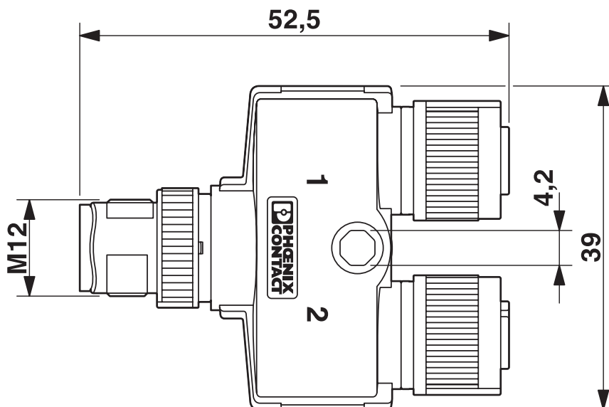
Rysunek wymiarowy
