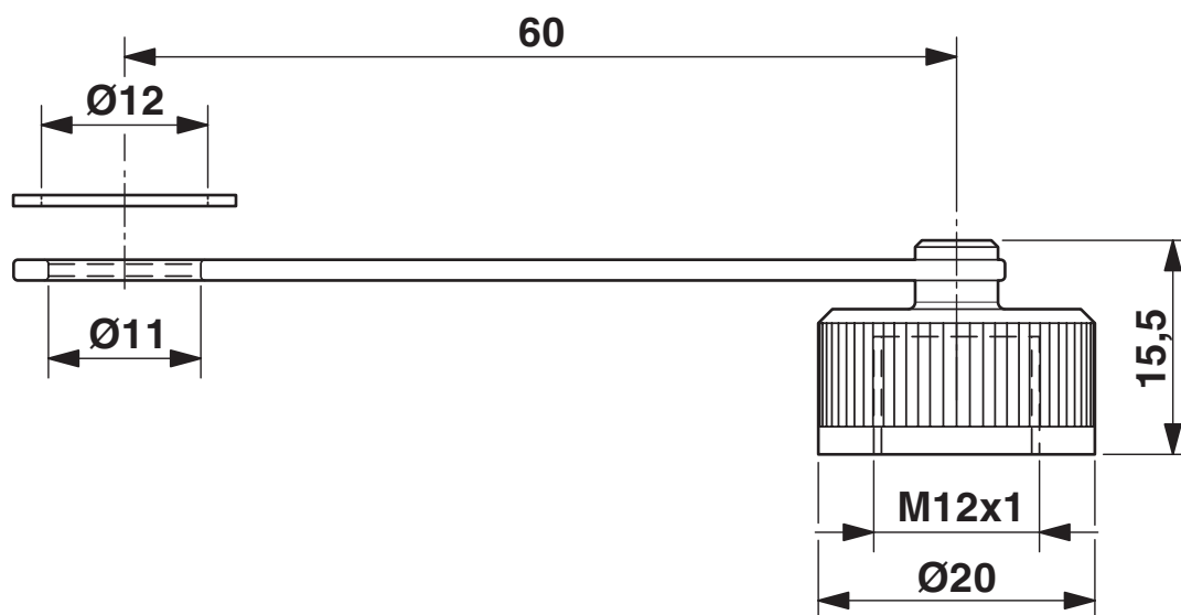
Rysunek wymiarowy
