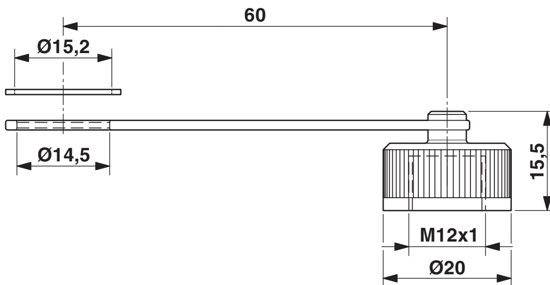
Rysunek wymiarowy
