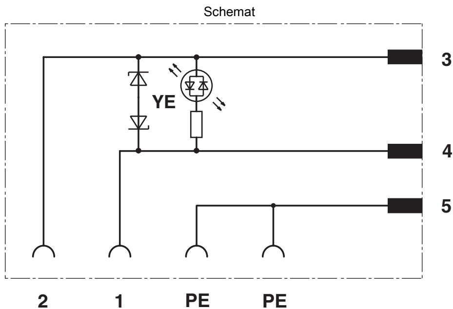
Rysunek schematyczny
