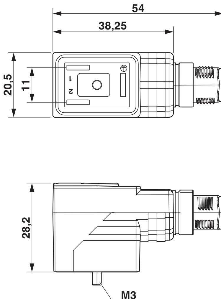
Rysunek wymiarowy
