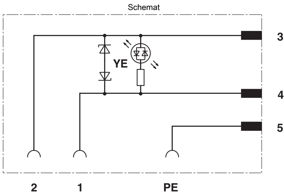
Rysunek schematyczny
