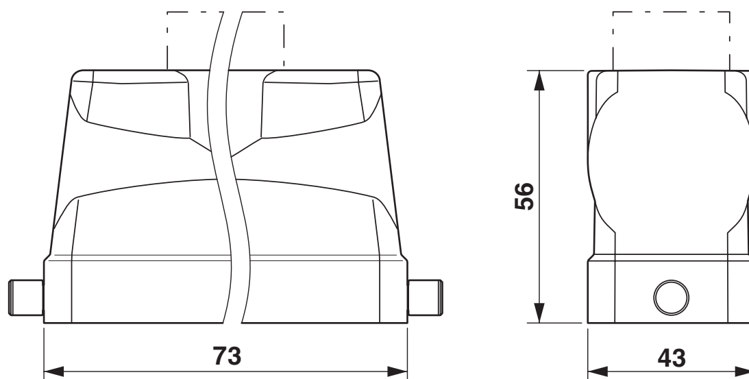
Rysunek wymiarowy
