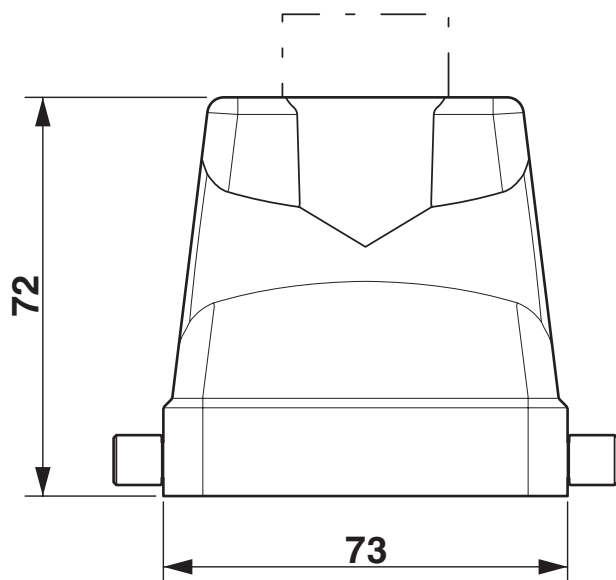
Rysunek wymiarowy
