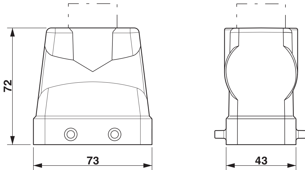
Rysunek wymiarowy
