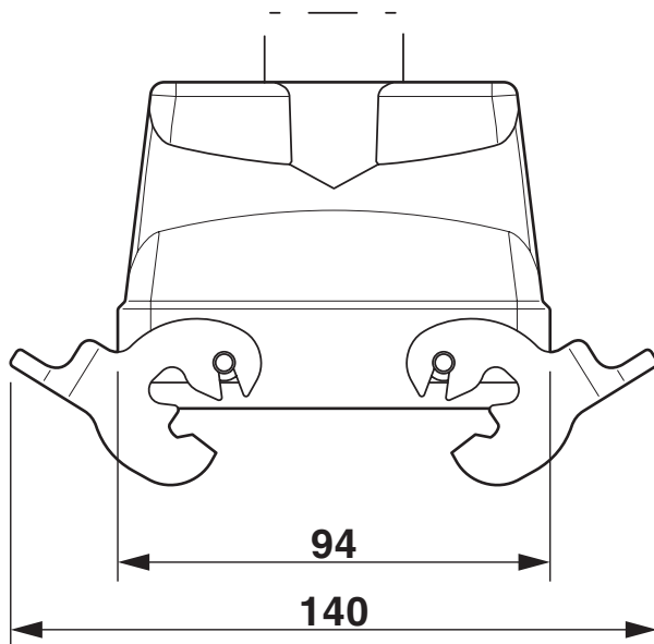
Rysunek wymiarowy
