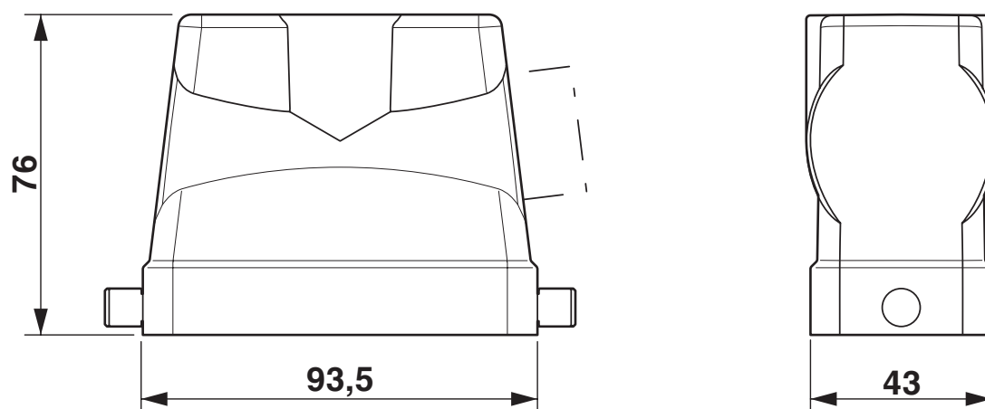
Rysunek wymiarowy
