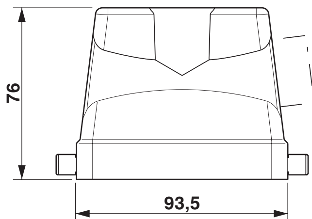
Rysunek wymiarowy
