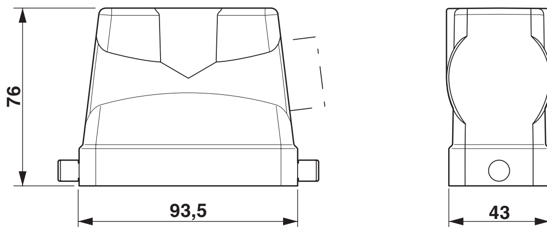
Rysunek wymiarowy
