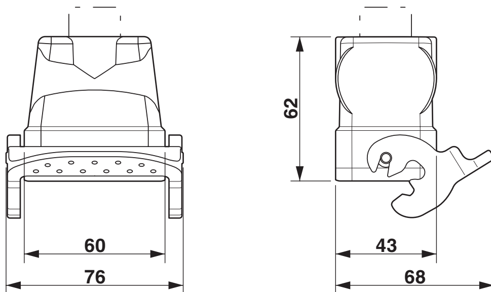
Rysunek wymiarowy
