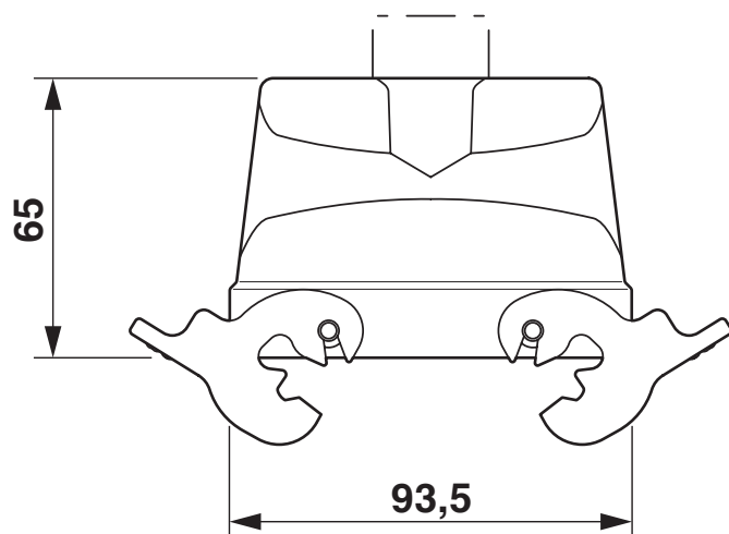
Rysunek wymiarowy
