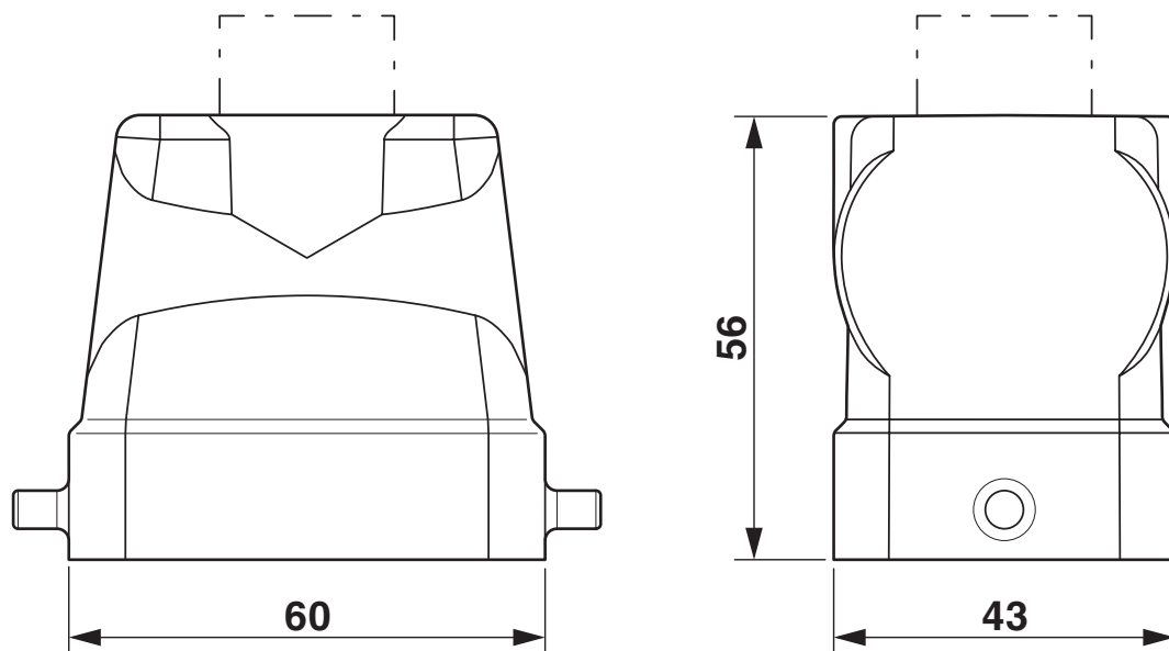
Rysunek wymiarowy
