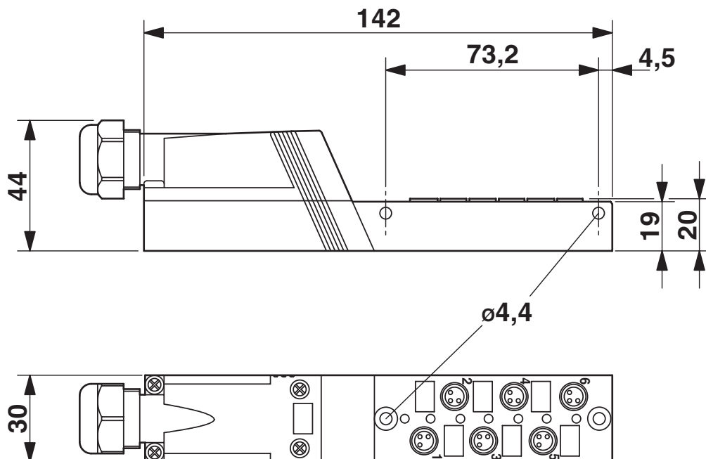
Rysunek wymiarowy
