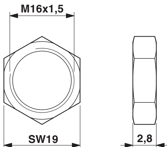
Rysunek wymiarowy
