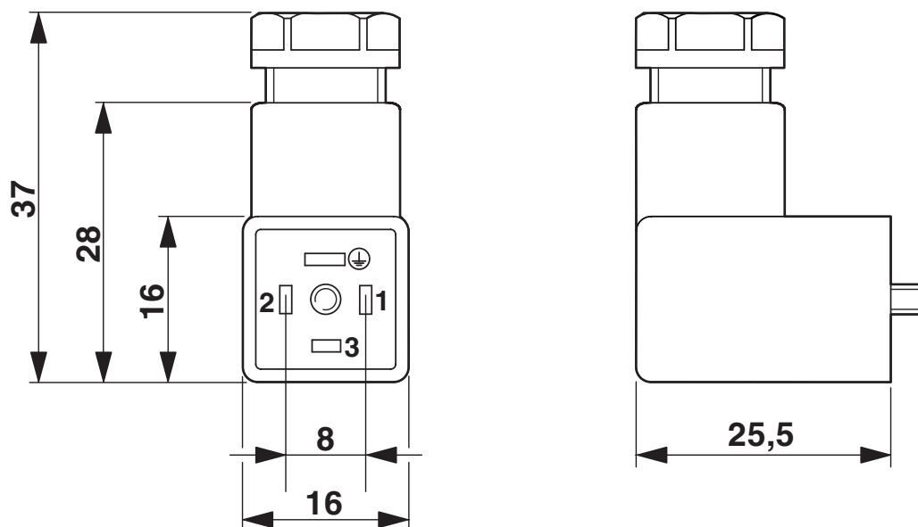
Rysunek wymiarowy
