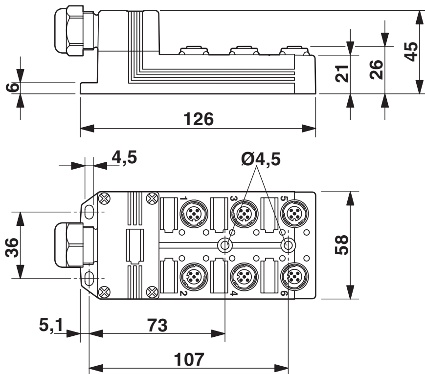
Rysunek wymiarowy
