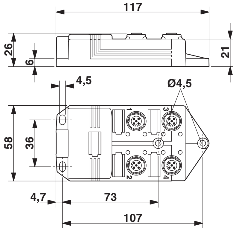
Rysunek wymiarowy
