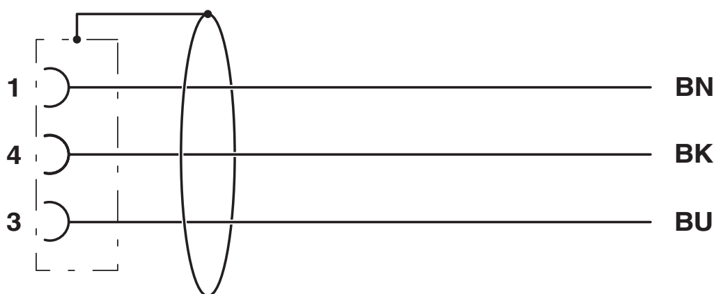
Schemat
