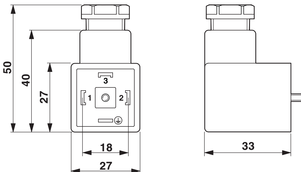
Rysunek wymiarowy
