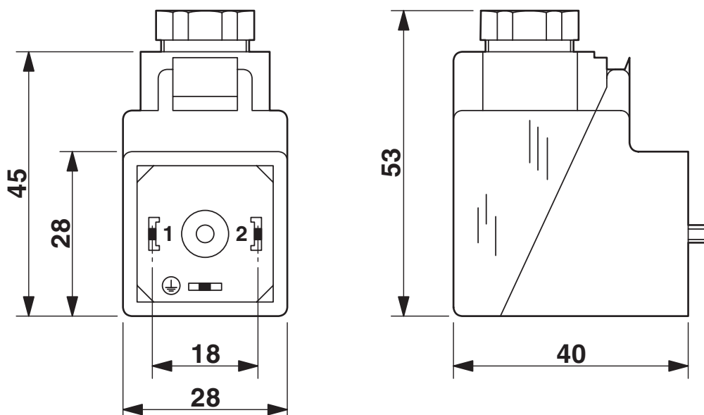
Rysunek wymiarowy
