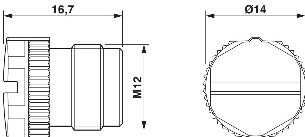
Rysunek wymiarowy
