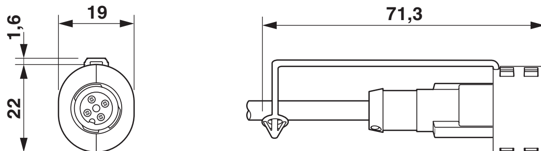
Rysunek wymiarowy
