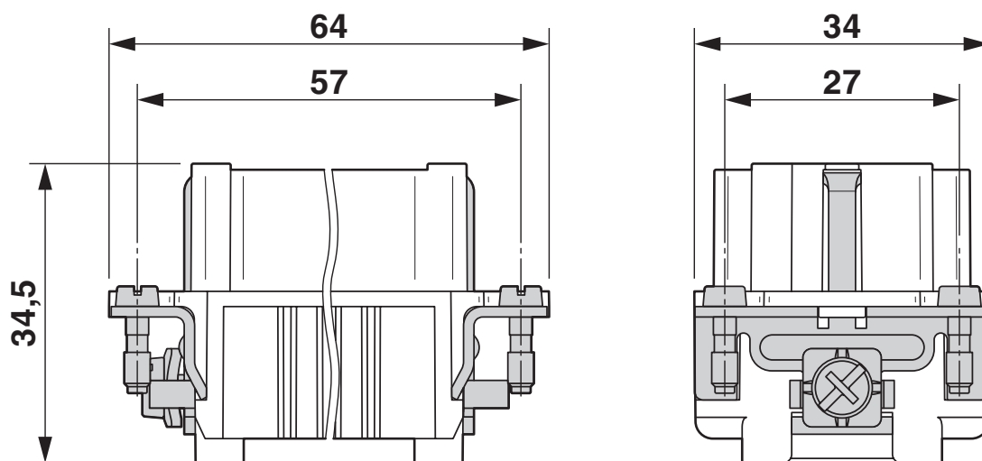
Rysunek wymiarowy
