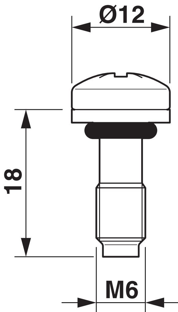
Rysunek wymiarowy
